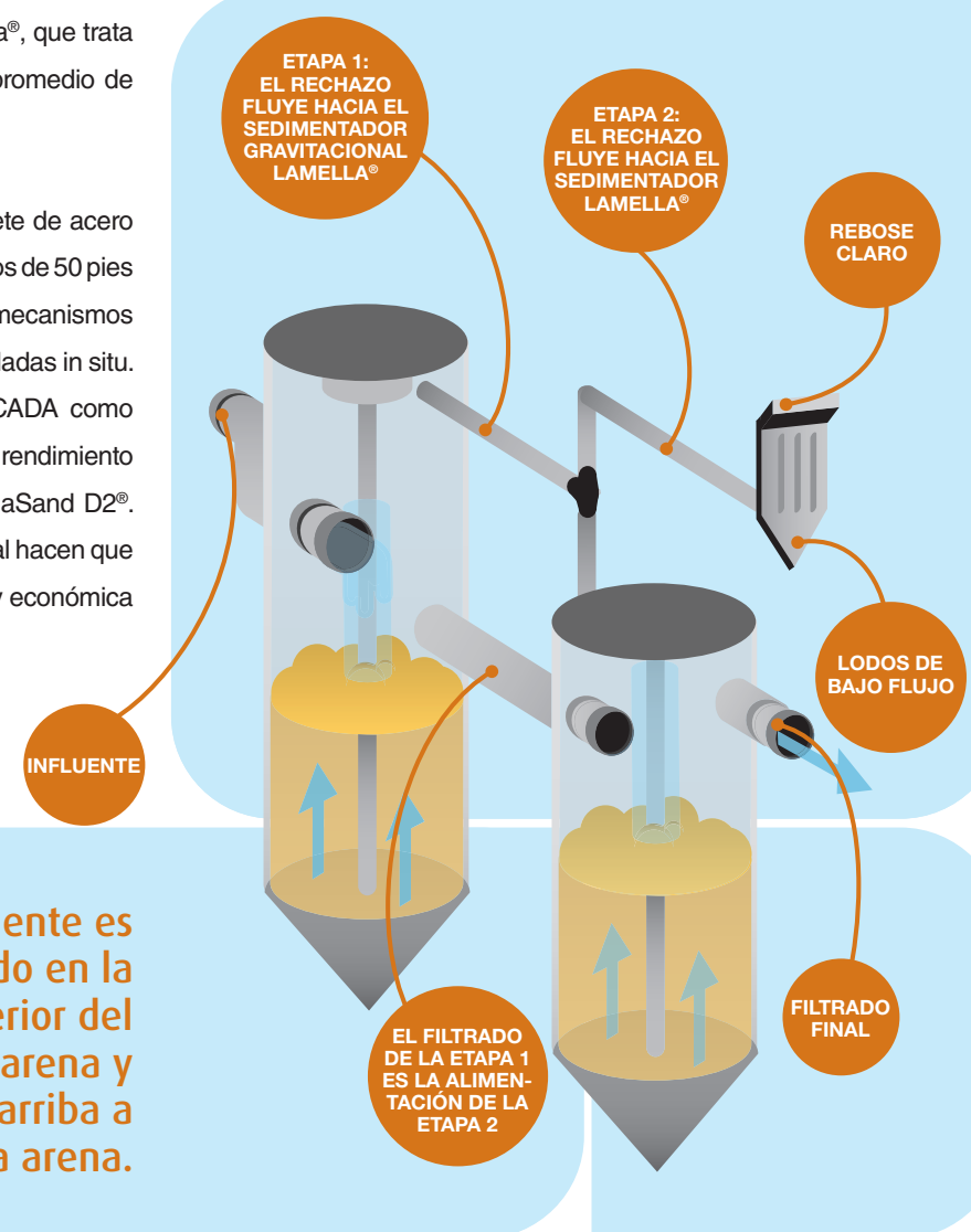
Dentro de un Filtro Dynasand®
